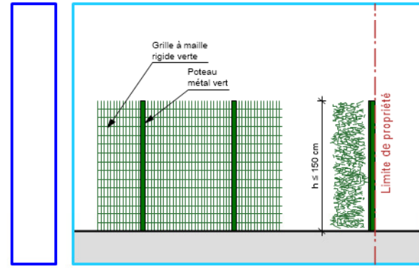
Clôture type 1 en périphérie de l'opération et en limite entre les lots
