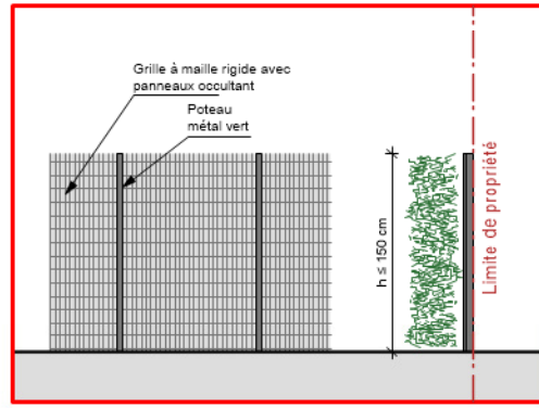
Clôture type 2 en périphérie des lots
