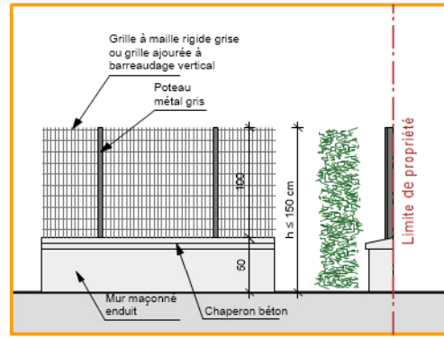
Clôture type 3 en limite des espaces publics pour les lots à bâtir
