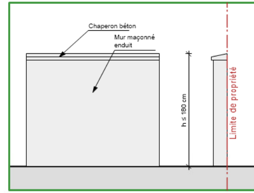
Clôture type 4 en limite entre les lots (si accord du mitoyen)
