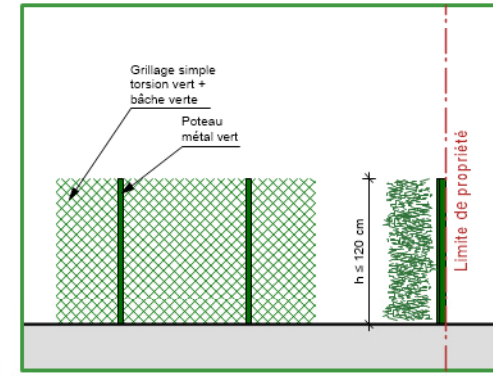
Clôture type 5 en limite entre les lots
