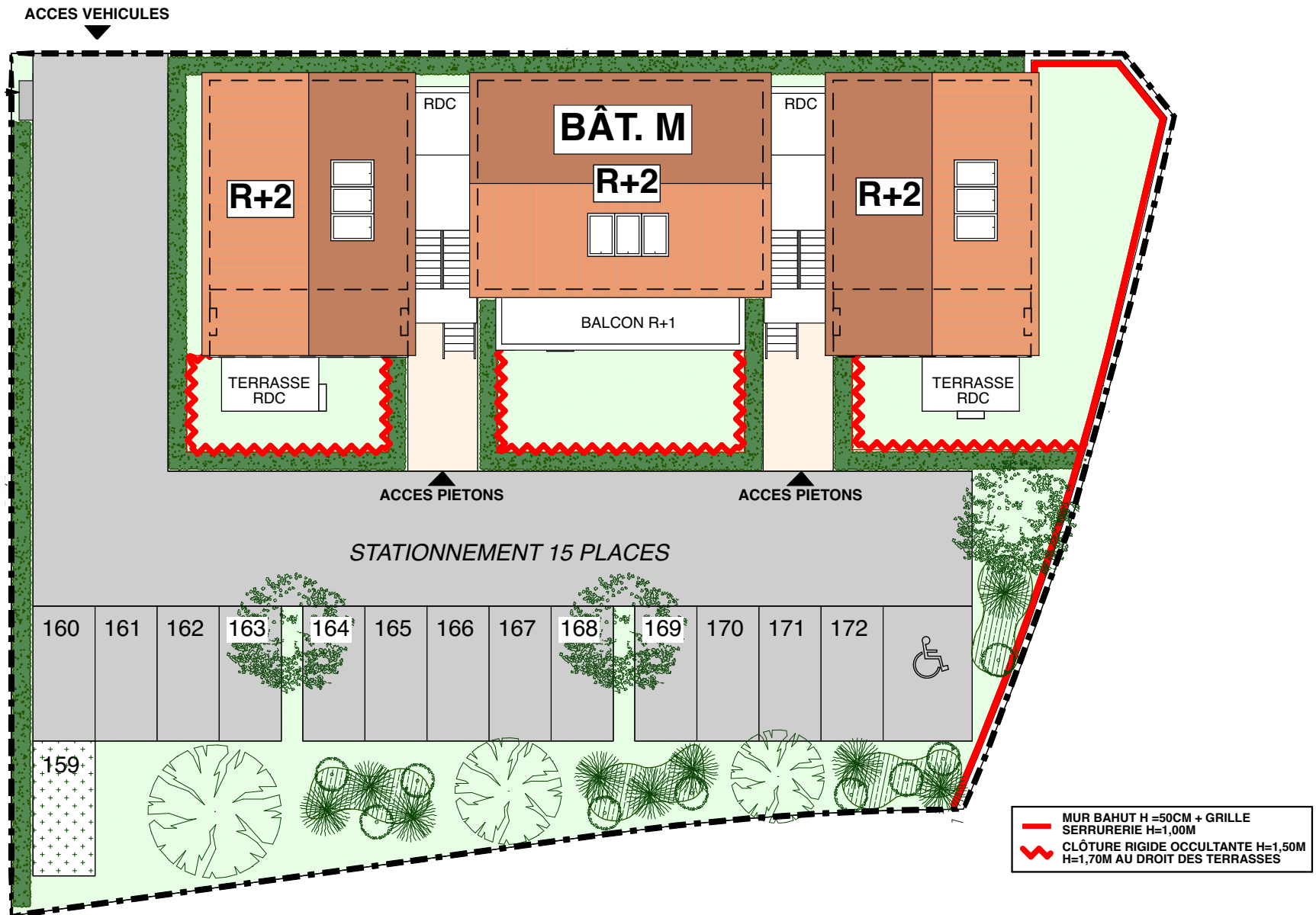
PLAN DE MASSE – MACROLOT N°09
