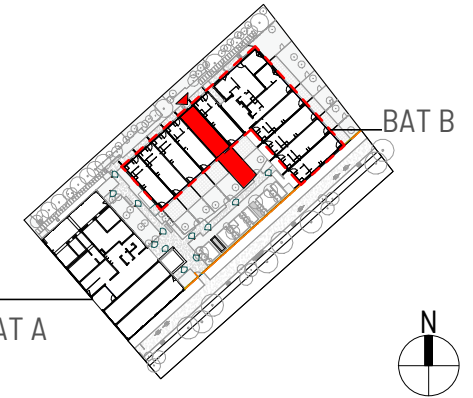
BAT B / Appartement n°23 / T3 / RDC
