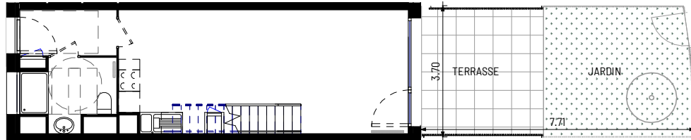
REZ-DE-CHAUSSÉE_PLAN DE JARDIN_150e
