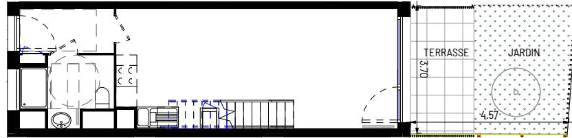
REZ-DE-CHAUSSÉE_PLAN DE JARDIN_150e
