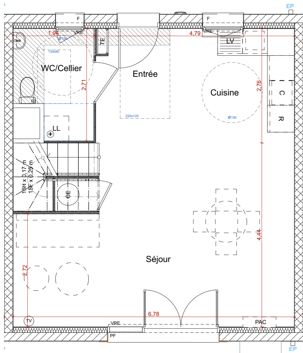
PLAN RdC
