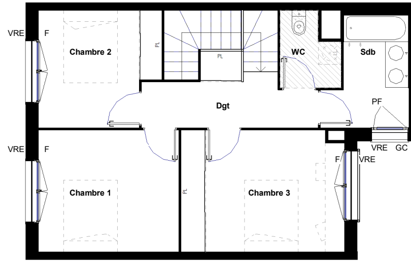
ETAGE 1
