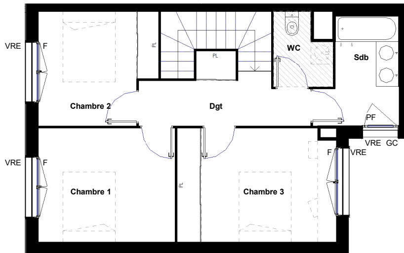
ETAGE 1
