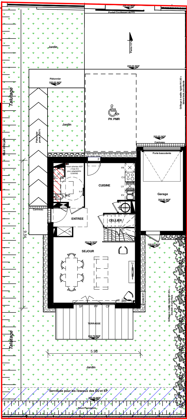
REZ DE CHAUSSEE
